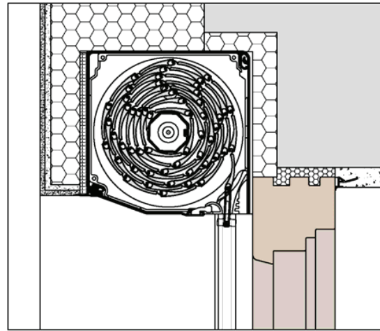
Sturzdämmung bauseits
